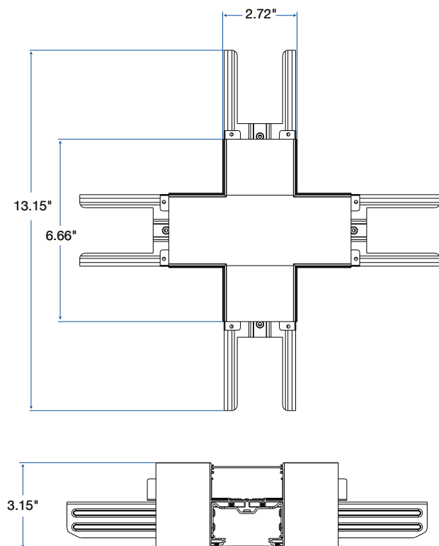
Connecteur (X) ALV-CON-X-XX
