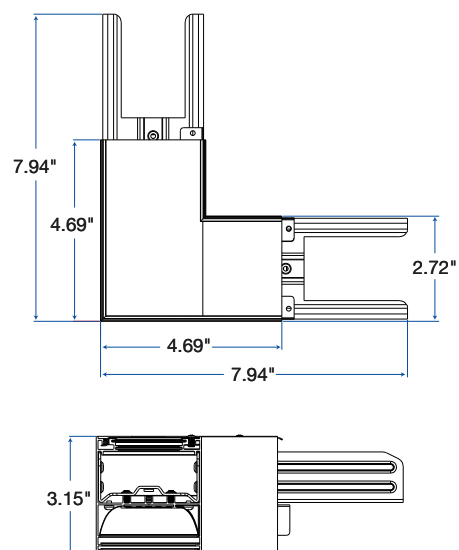
Connecteur (L) ALV-CON-L-XX
